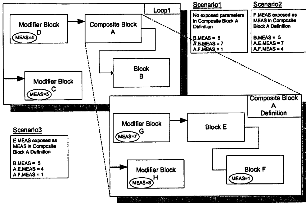
Figure 86 - Modifier Block Parameter override precedence
